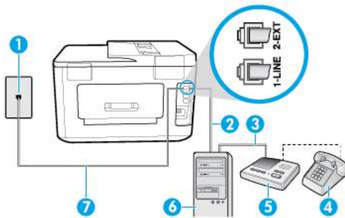
Figura 5-13 Vista posterior de la impresora
